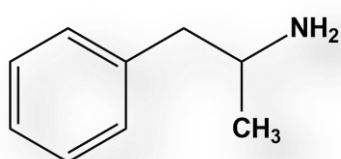
Anfetamina 1-Fenilpropan-2-amina
