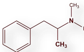
Metanfetamina N -metil-1-fenilpropan-2-amina
